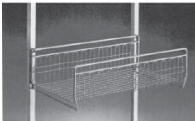
Para Esterilizadores Dim.: 560x310x170mm 36282-00
