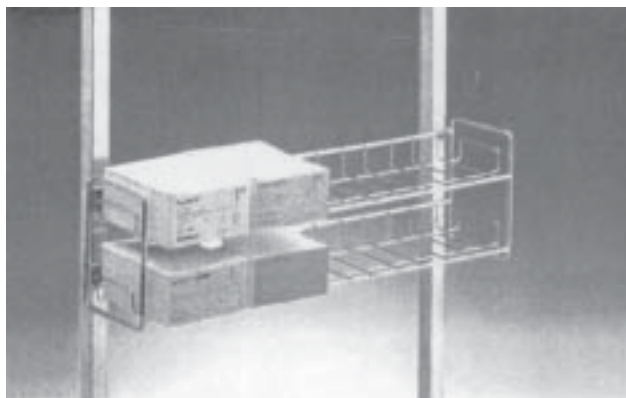
Para Suturas Dim.: 580x140x200mm 36271-00
